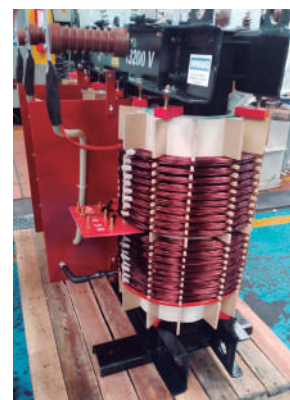
Transformador de 500KVA para su instalación
